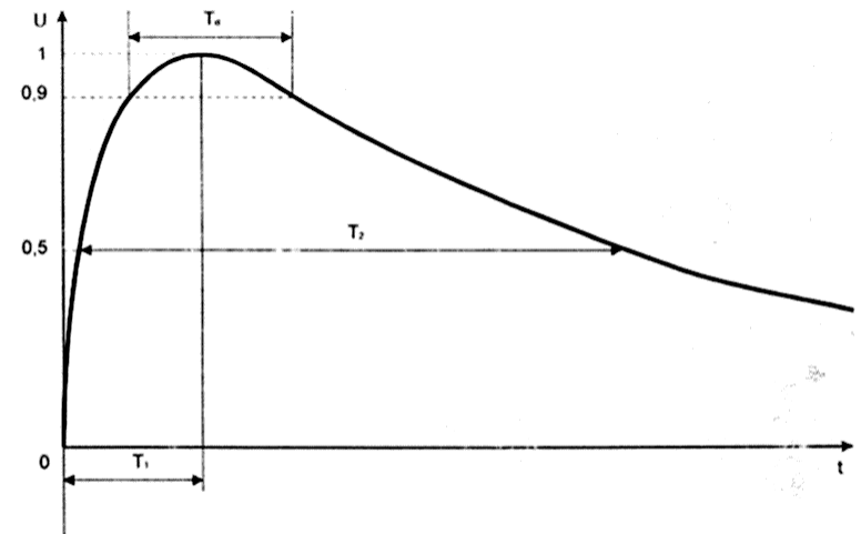
Onda de sobretensión tipo maniobra 250/2500 \mu\text{s} normalizada según UNE 21308.
