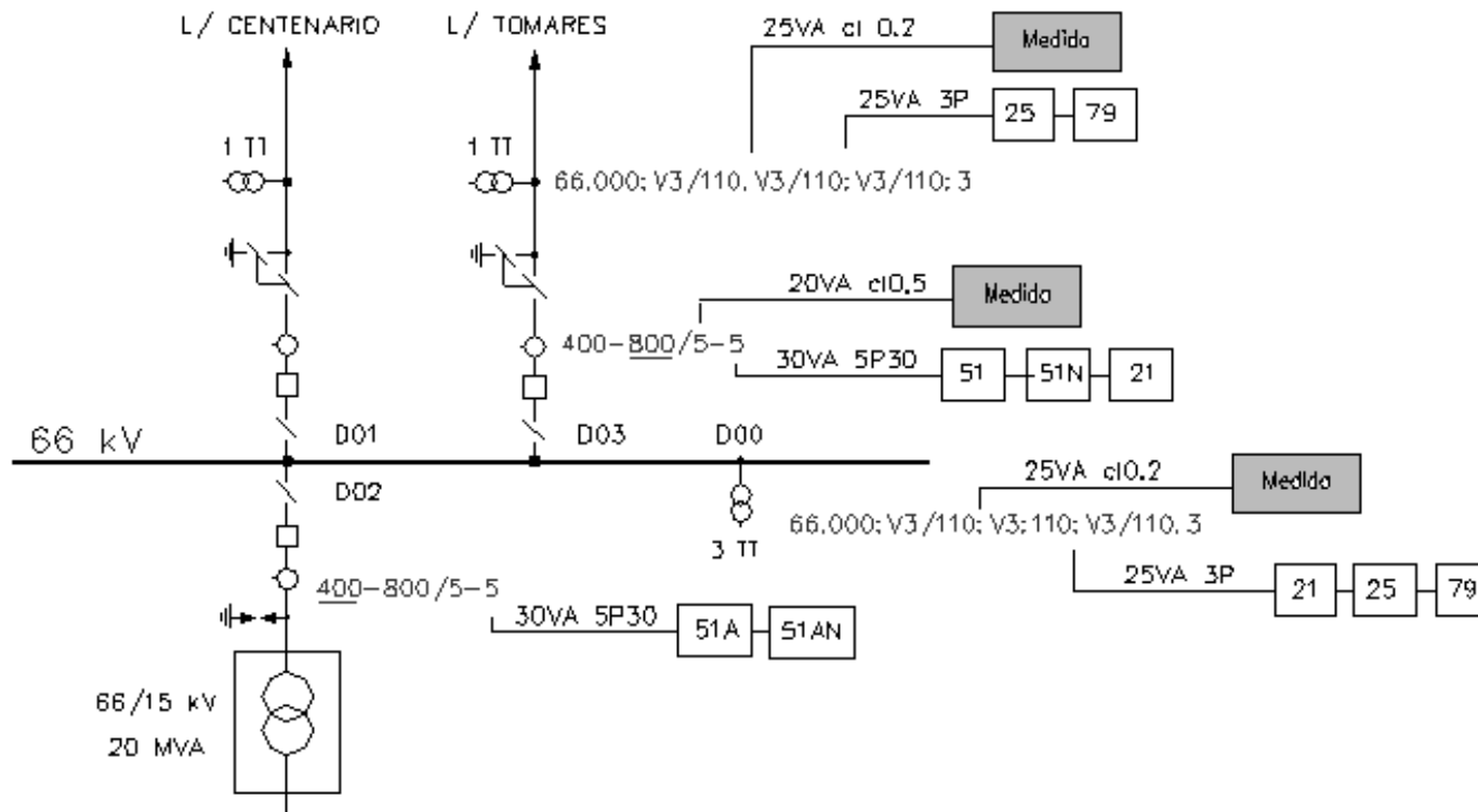
Puntos de medida en S/E 66/15 kV
